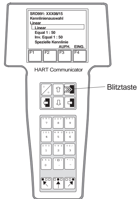
Beispiel für eine Menüanzeige auf der Handterminal-Bedienoberfläche: Untermenü "Kennlinienauswahl" (2.3.1.4.9.) 2)
